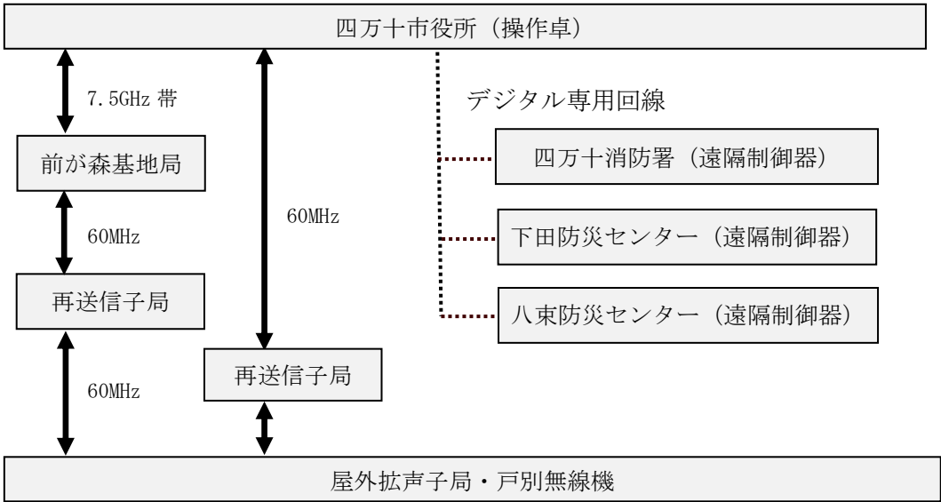
システム系統図
