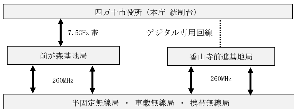
システム系統図
