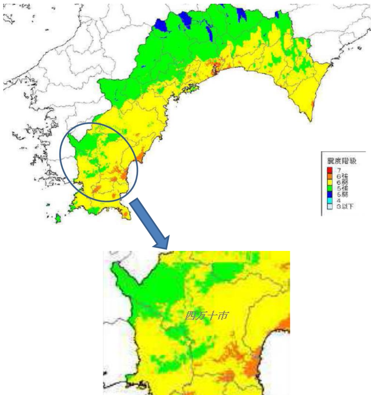
震度分布図
