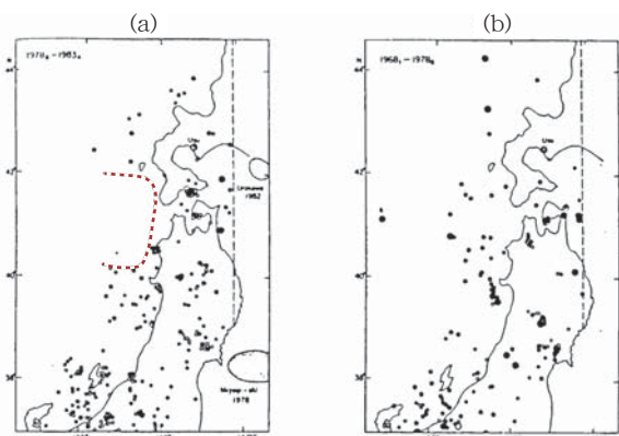
図1 1983年日本海中部地震の直前5年間に現れた「第2種空白域」(茂木清夫, 1983)
