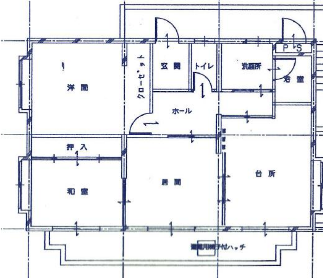
(1) 間取図
