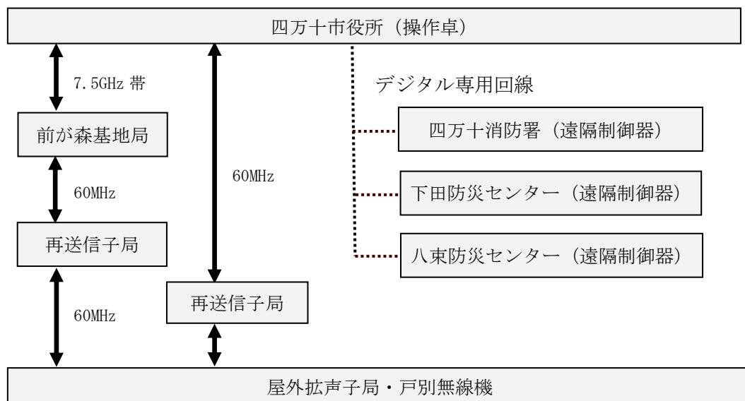
システム系統図
