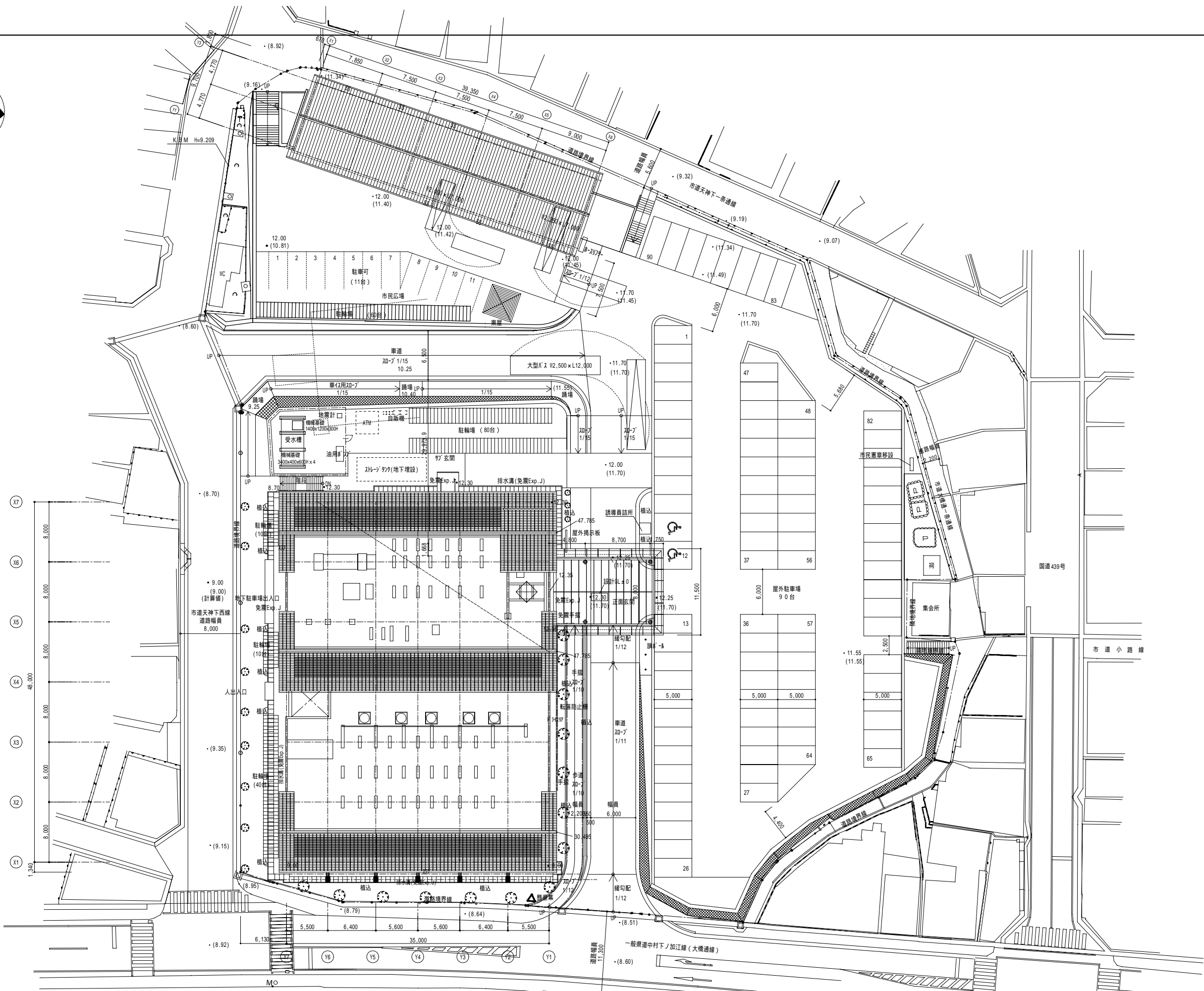
配置図 1/250
